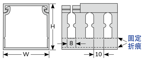
出线孔尺寸
