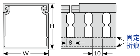
出线孔尺寸
