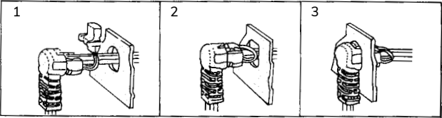
电源线扣装配图
