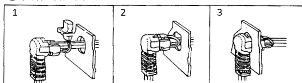
电源线扣装配图
